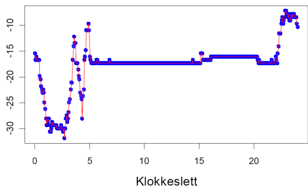
Vertikalvandringsdiagram
