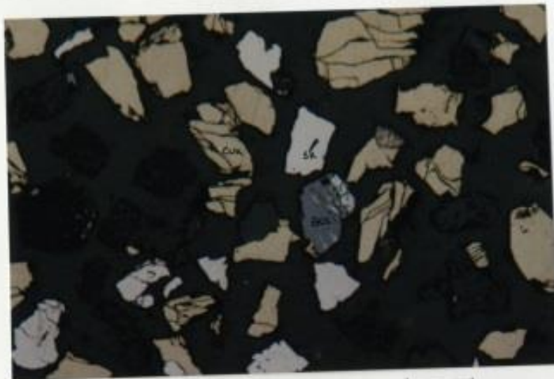
Kuva 14. Bidjovagge, Norja; rikaste +74 \mu\text{m} 2-4.10.86 (P13523). Pyriittiä (SK) ja sinkkivälkettä (ZNS) rikasteessa. Suurennus 175x.
