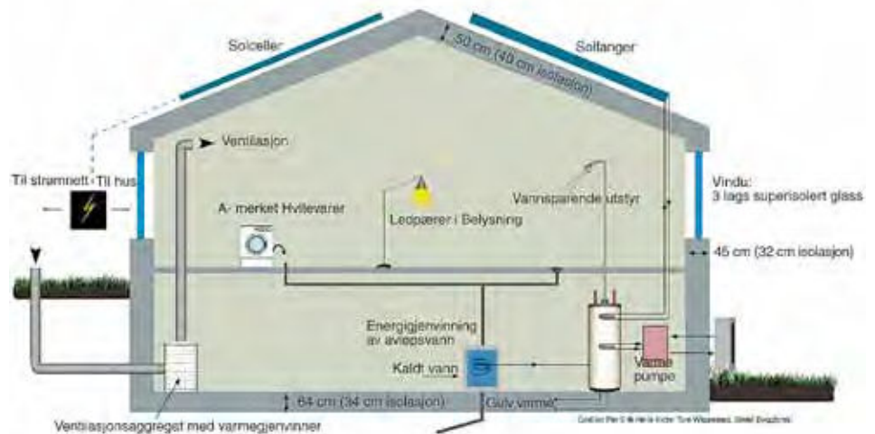
Et passivhus har tykkere isolasjon, kontrollert ventilasjon med varmegjenvinning og spesielt energieffektiv belysning og utstyr.
