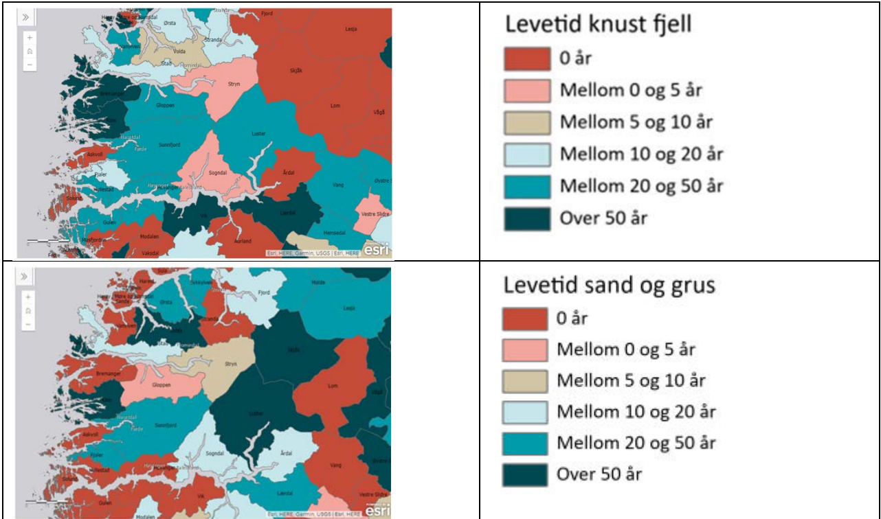
Figur 3.5. DMFs levertidskart for henholdsvis knust berg (a) og sand og grus (b), viser hvor mange år hver enkelt kommune vil ha tilgang på egenprodusert knust fjell, sand og grus før de går tom for ressurser [21, 22].
