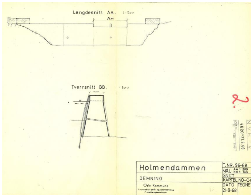
Figur 2: Snitt-tegning Holmendammen. Damkronen er innmål på ca. kote 112,17, mens overløpsterskelen ligger på ca. kote 111,43.
