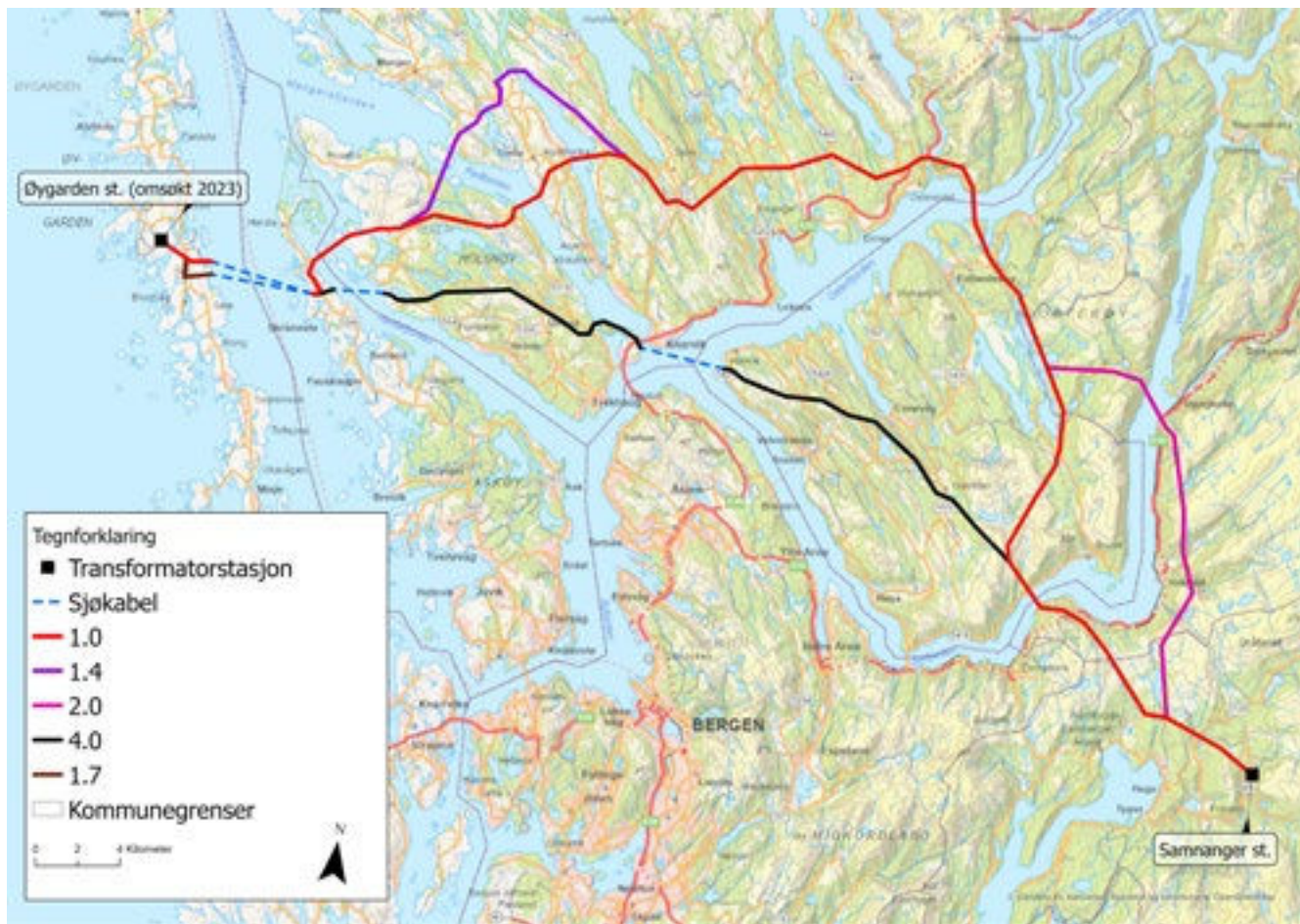
Oversikt over meldte alternativer for ny 420 kV forbindelse mellom Samnanger transformatorstasjon og ny Øygarden transformatorstasjon.
