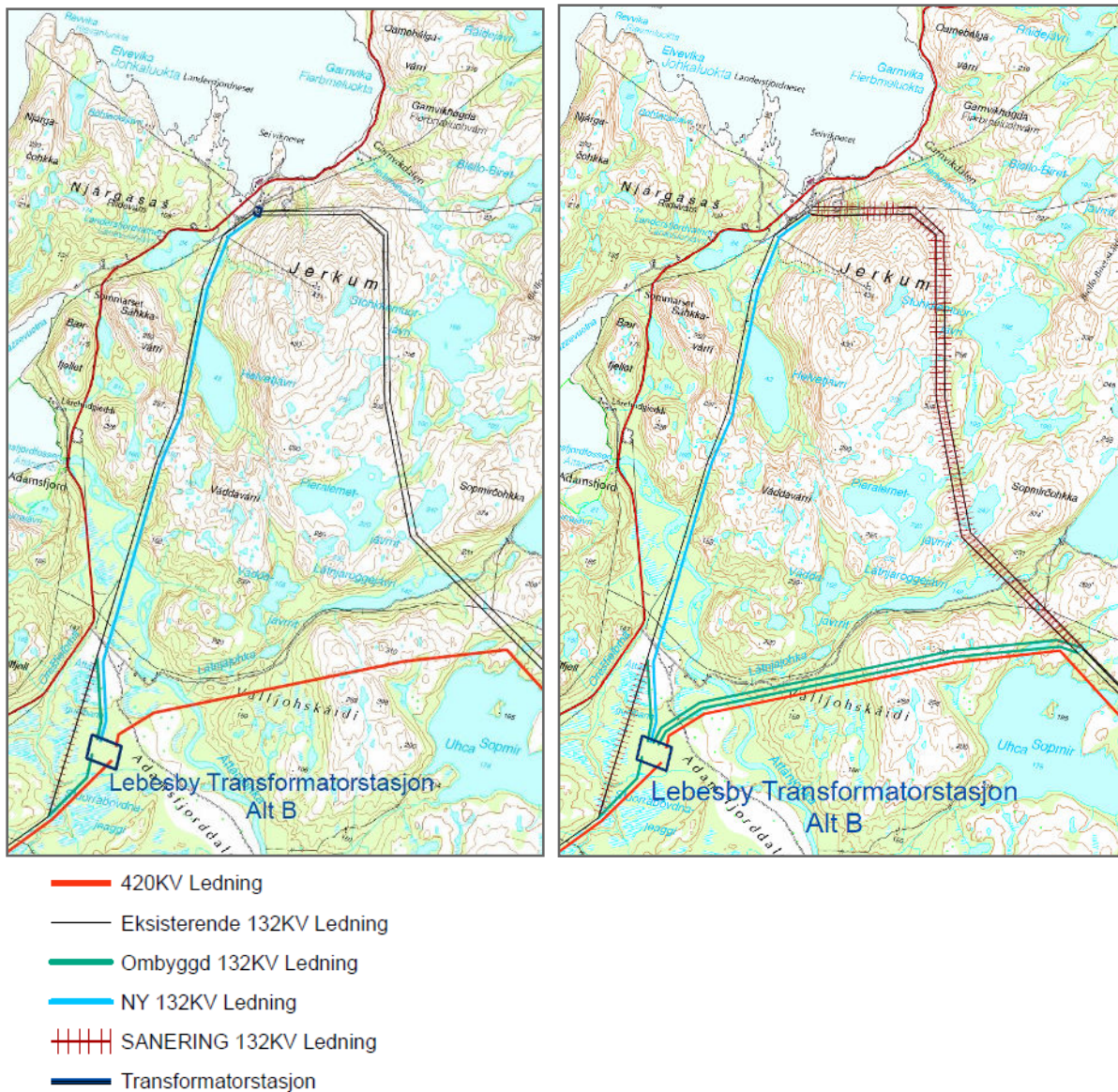
Figur 12: Kartene viser et par alternative løsninger for ledningsføringer ved valg av stasjonalternativ B i Lebesby. Planlagt ny 420 kV-ledning er vist med rød strek. Mellom ny stasjon og dagens Adamselv stasjon er det planlagt en 132 kV-ledning i tillegg til den som går der i dag. Dagens 132 kV-ledninger er vist med sort strek. Kartet til venstre viser en løsning der dagens ledninger beholdes som i dag. Til høyre et alternativ der dagens ledninger fra Adamselv mot Varangerbotn og Tana bru legges inn til ny stasjon i stedet for til Adamselv. Mulighetene for å rive en eller flere av dagens 132 kV-ledninger når ny ledning er på plass, vil bli utredet.
