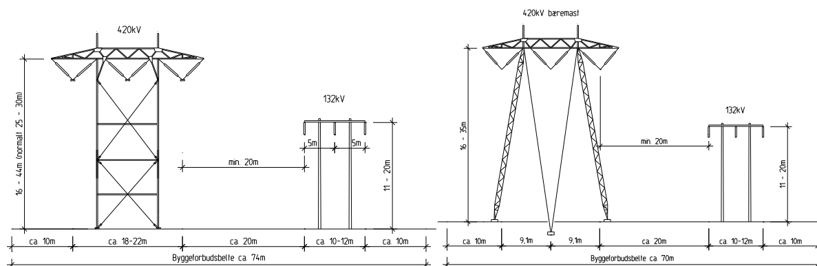
Figur 6: Mastebilde ved parallellføring med eksisterende 132 kV trestolpeledning. Til venstre ved bruk av selvbærende mast, og til høyre med utvendig bardundert mast. Bredden på ryddegaten og byggeforbudsbeltet blir da ca 70m.
